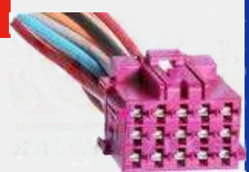
CONECTOR QUINCE VÍAS HEMBRA ROSADO
